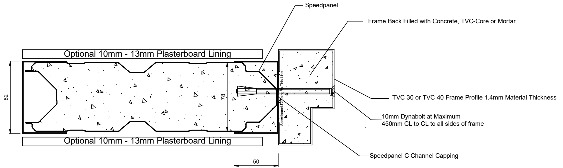
FIRECORE TVC-30 (FRS58)
